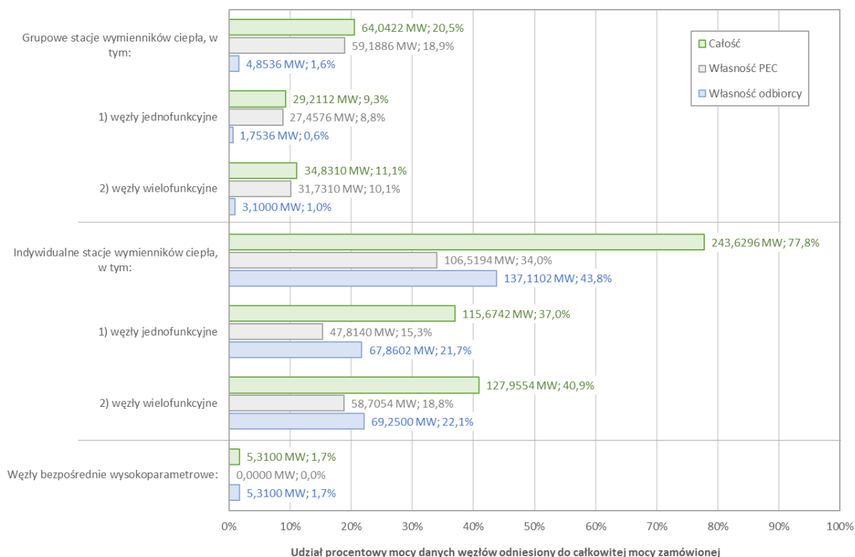
Rysunek 8. Moc zamówiona obsługiwanych węzłów ciepłych w roku kalendarzowym (stan na 31.12.2024 r.), z rozdziałem rodzajowym węzła
