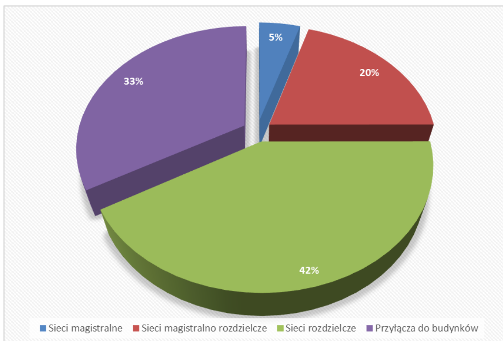
Rysunek 3. Charakterystyka zbiorcza sieci ciepłowniczej – podział sieci ciepłowniczej ze względu na jej rodzaj / funkcję
