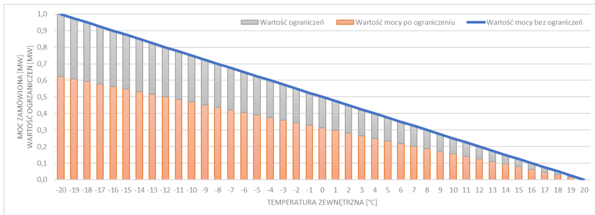
Rysunek 17. Zmienność jednostkowej mocy zamówionej o wartości 1MW w warunkach szczytowych względem temperatury zewnętrznej dla układu ogrzewczego do utrzymania temperatury w pomieszczeniu na poziomie 10°C
